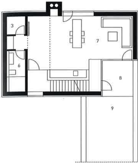
Obergeschoss M 1:200
